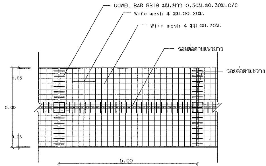
แปลนแสดงการเสริมเหล็กถนน คลล. NOT TO SCALE
