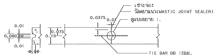
แบบขยาย 1. NOT TO SCALE
